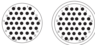
Gehäuse 2 37 x ø 1 mm
