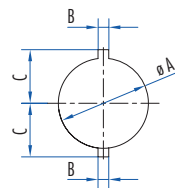
Abb. 2: Wandstärke über 10 mm
