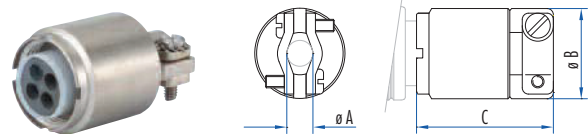
Kabelklemme für Natto Miniatur Push-Pull
