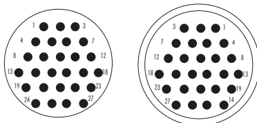
Gehäuse 2 27 x ø 1 mm
