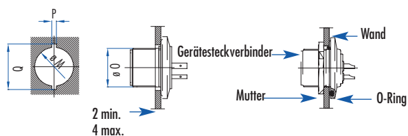
Abb. 1: Wandstärke zwischen 2 und 4 mm
