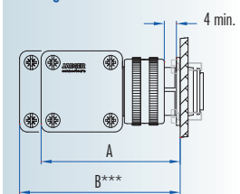
Montage Kabelsteckverbinder – Gerätesteckverbinder
