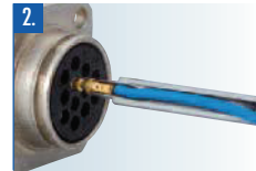
2. Den Draht und den gecrimpten Kontakt in der Rinne dieses Trägers positionieren. Die Einheit gemäß dem Verkabelungsplan hinter dem Geräte- oder Kabelsteckverbinder einführen, dabei in der Mitte des Isolierkörpers beginnen und nach außen zu der Stelle vordringen, die für die Aufnahme des Kontaktes vorgesehen ist. So lange drücken, bis der Träger am Anschlag ist. Den Träger entfernen. Die korrekte Platzierung der Kontakte durch leichtes Ziehen an jedem Draht prüfen.
